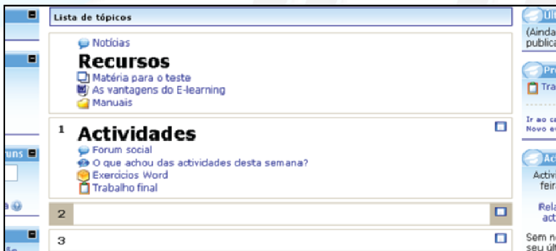
Figura 12 -Disciplina Tópicos
